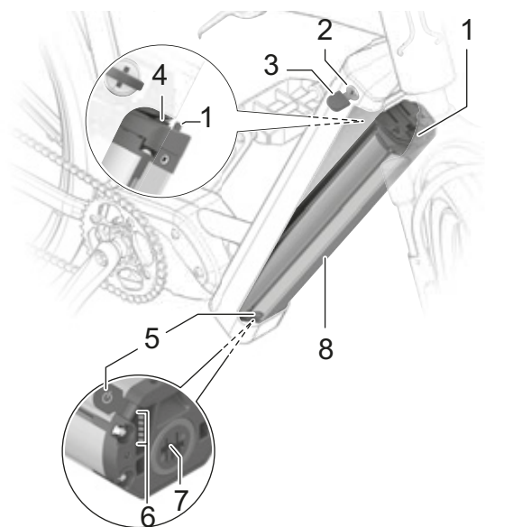
Illustration 36 : Détail de la batterie PowerTube 750
