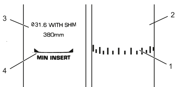
Illustration 74 : Vue détaillée de la tige de selle, exemples de marquage de la profondeur d'insertion minimale
