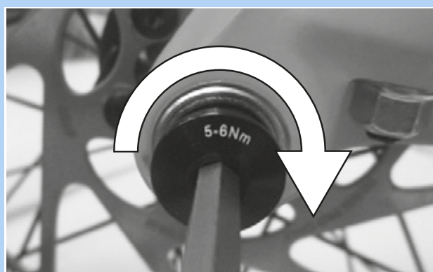
Illustration 55 : Serrer la vis de blocage
