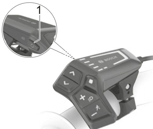
Illustration 120 : Position de la touche Marche/Arrêt sur le BOSCH LED Remote
