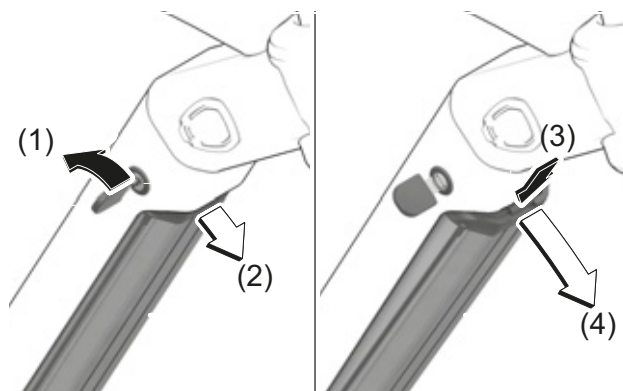
Illustration 118 : Retirer la batterie intégrée
