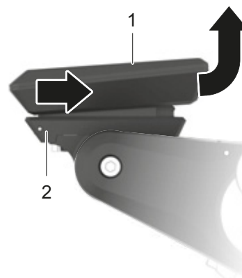
Illustration 109 : Retirer l'ordinateur de bord
