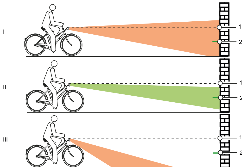
Illustration 139 : Feu réglé trop haut (1), correctement (2) et trop bas (3)
