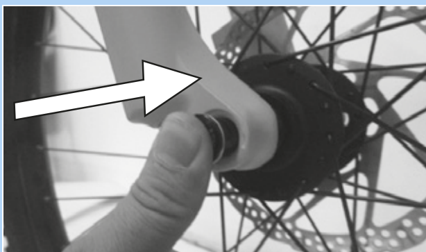
Illustration 52 : Enfoncez l'axe dans le sens de la flèche
