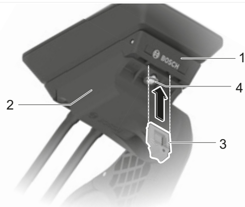
Illustration 108 : Position de la vis du jeu de direction
