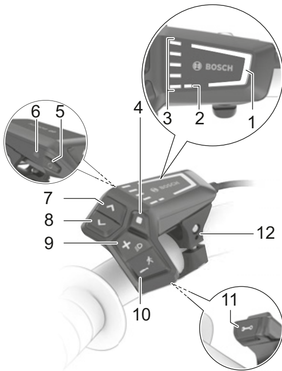
Illustration 110 : Aperçu de l'unité de commande BOSCH LED Remote
