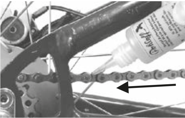
Illustration 133 : Lubrifier la chaîne
